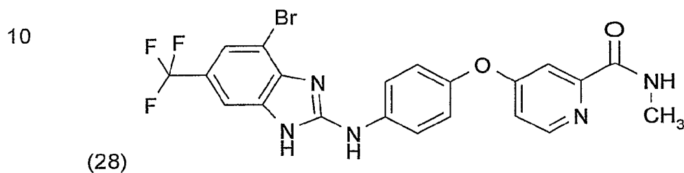
4-[4-(Brom-trifluormethyl-1H-benzimidazol-2-ylamino)-phenoxy]-pyridin-2-carbonsäure methylamid
